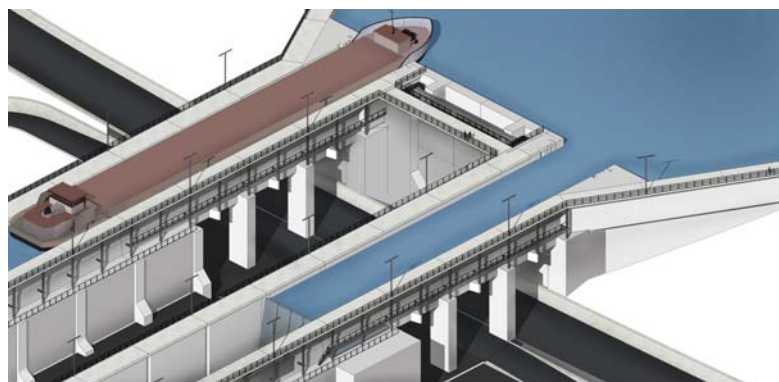
Detail průplavních mostů v horní části plavebních komor
