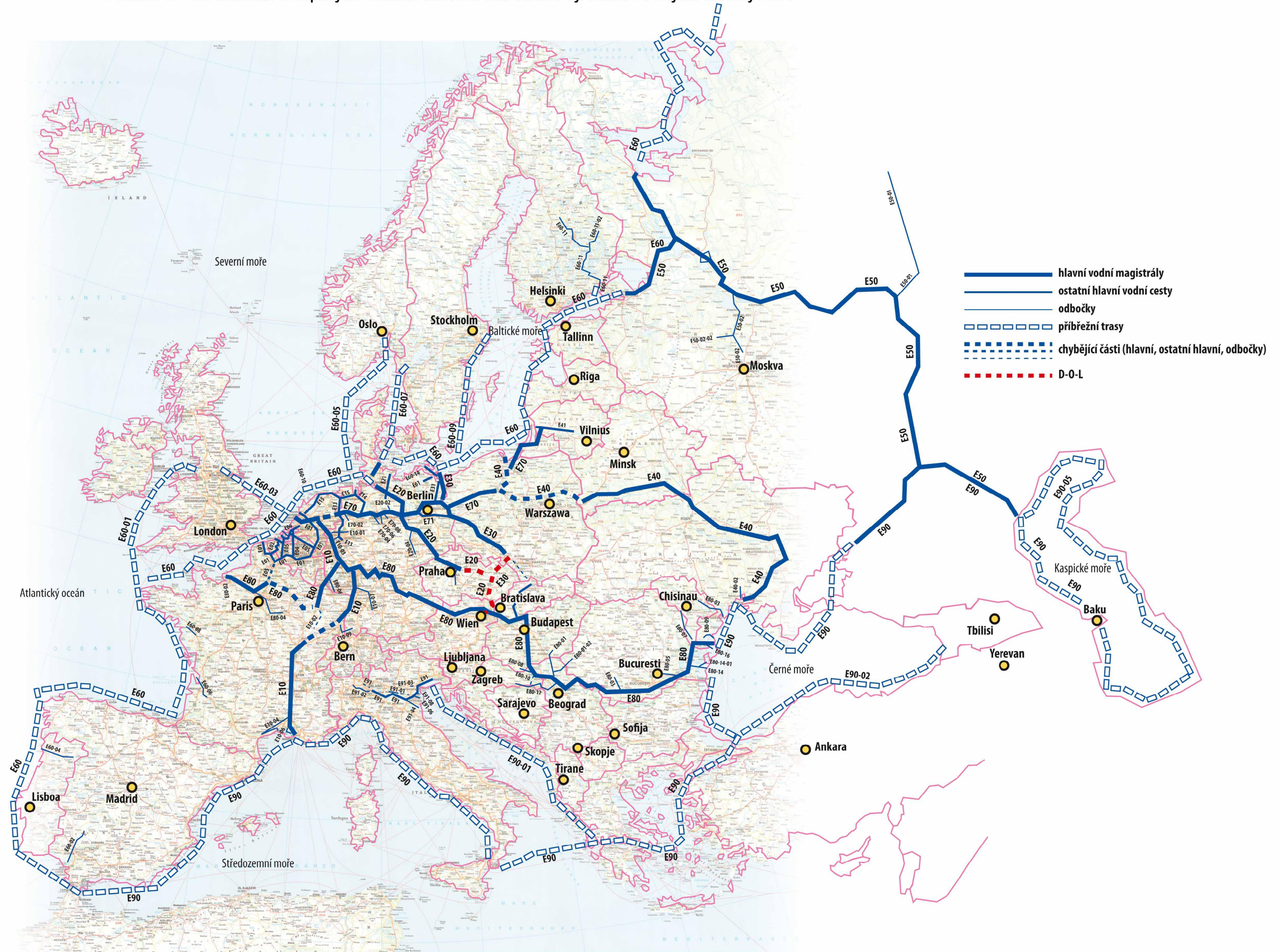
Příloha 1. - Síť hlavních evropských vodních cest mezinárodního významu ve smyslu dohody AGN
