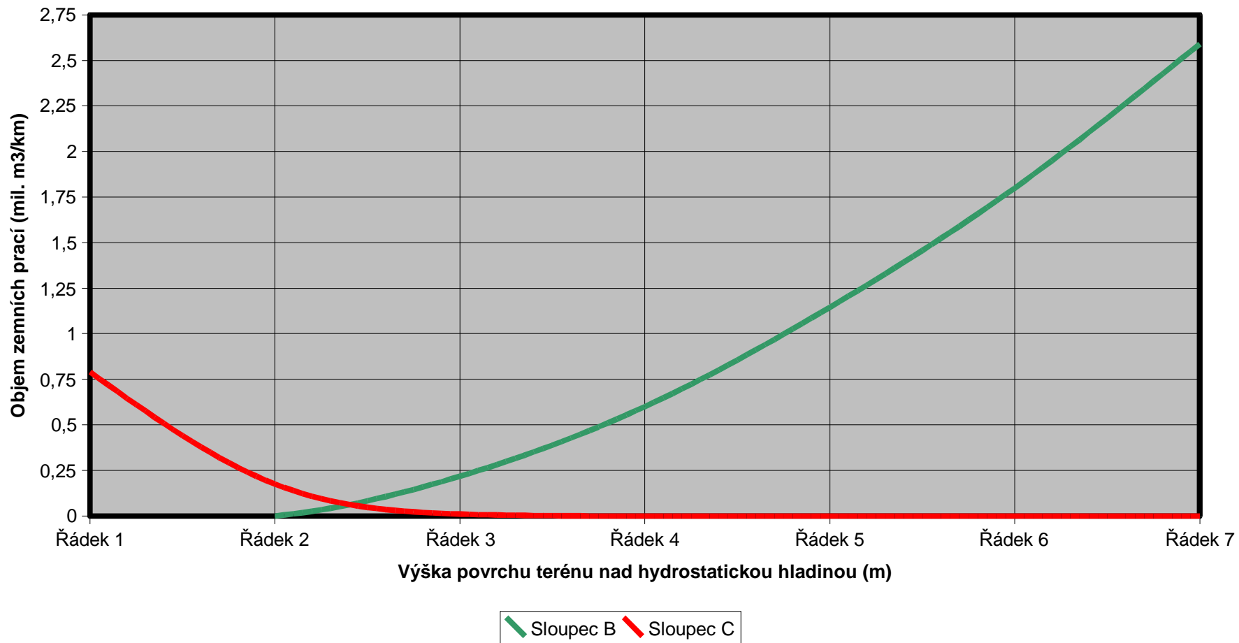
Příloha 6: Grafické určení objemu výkopů a násypů
